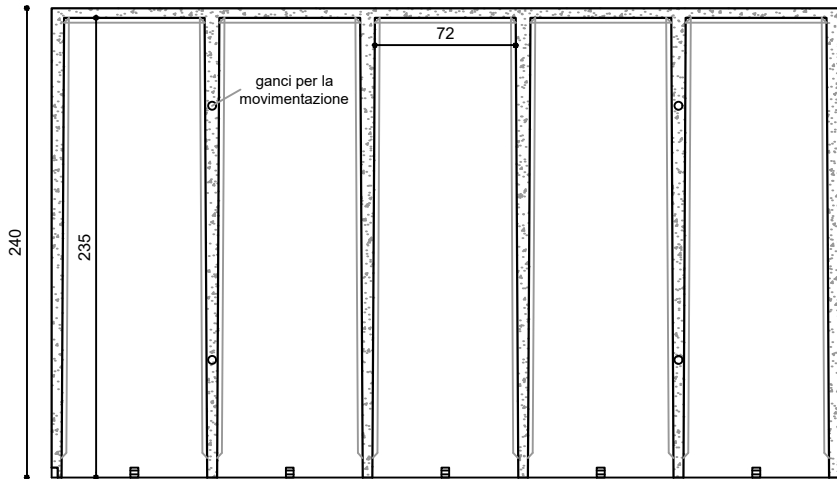
SEZIONE A-A'
