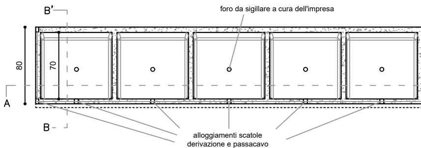
PROSPETTO
